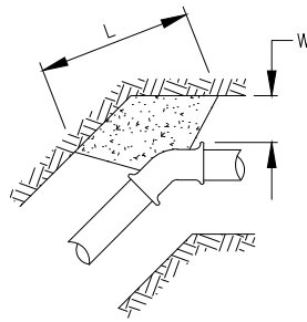
HORIZONTAL 45° BEND
